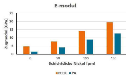
Abb. 1: E-Modul von PEEK und Polyamid
