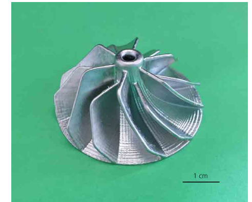
Abb. 1: Propellerrad, hergestellt über AM-Formgebung und Gelcasting
